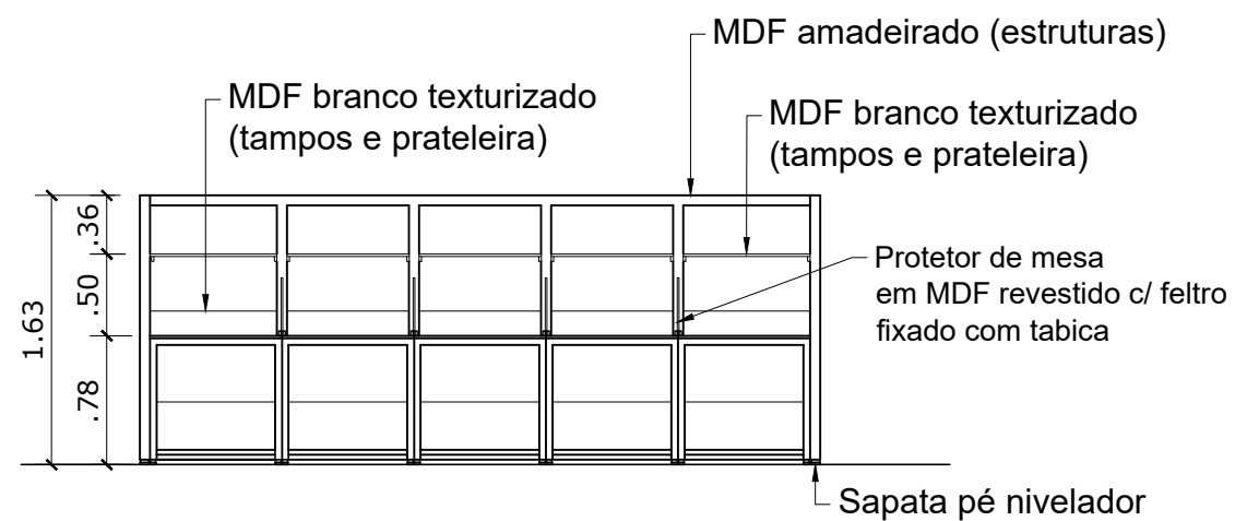
06 VISTA 02 - MOB. MODULAR ESC: 1/50
