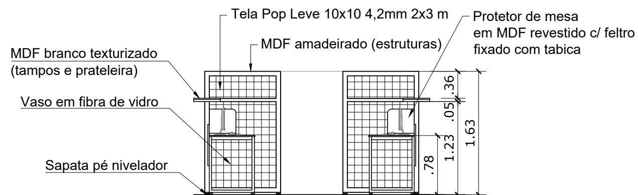
03 CORTE AA - MOB. MODULAR ESC: 1/50
