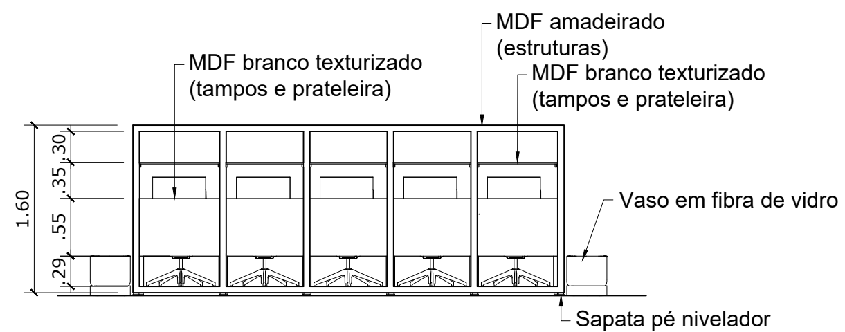
05 VISTA 01 - MOB. MODULAR ESC: 1/50
