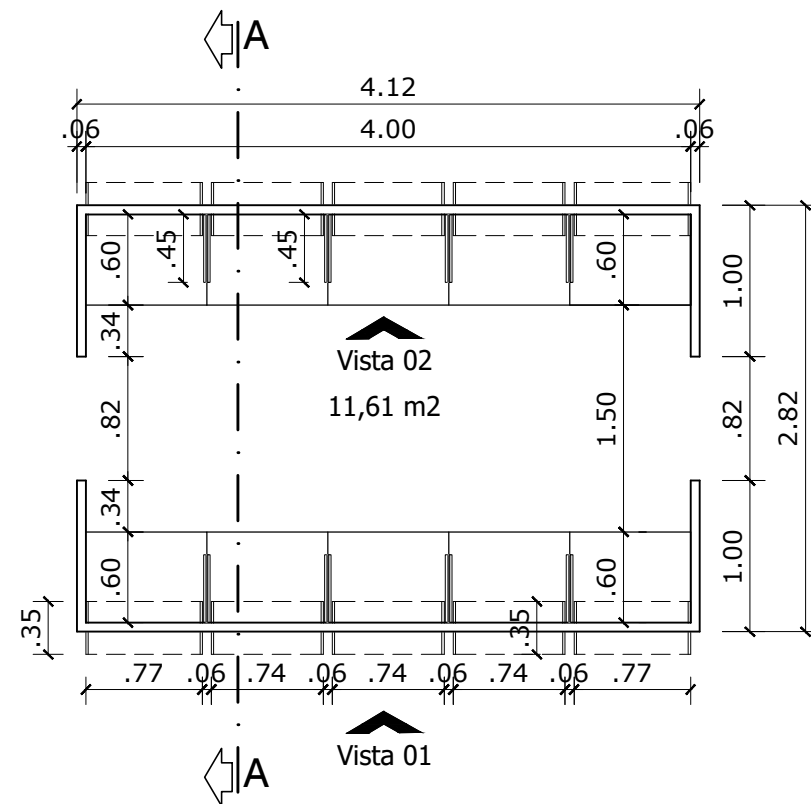
01 PLANTA BAIXA - MOB. MODULAR ESC: 1/50
